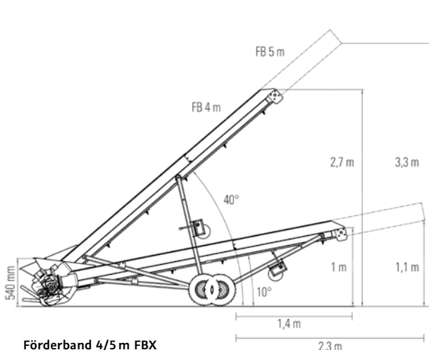
Förderband 4/5 m FBX Seitenansicht
